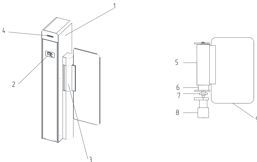
Рисунок 1 – Структура турникета:
