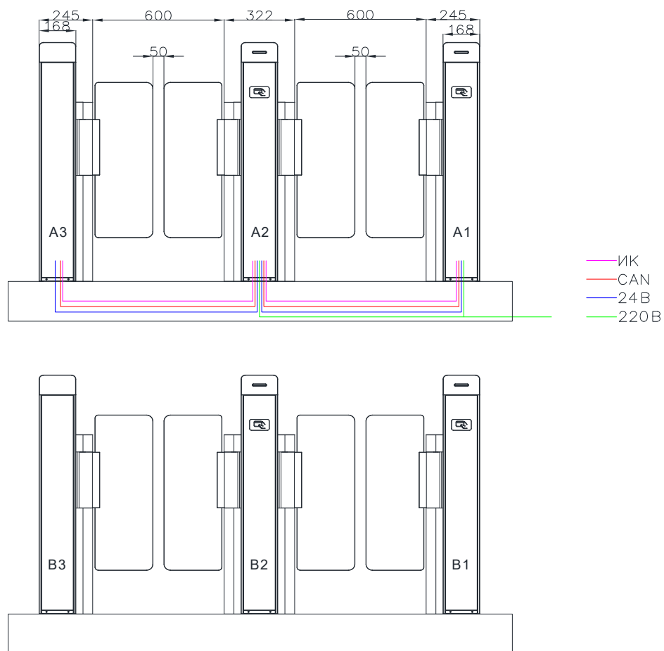
Рисунок 2 – Схема установки турникета
