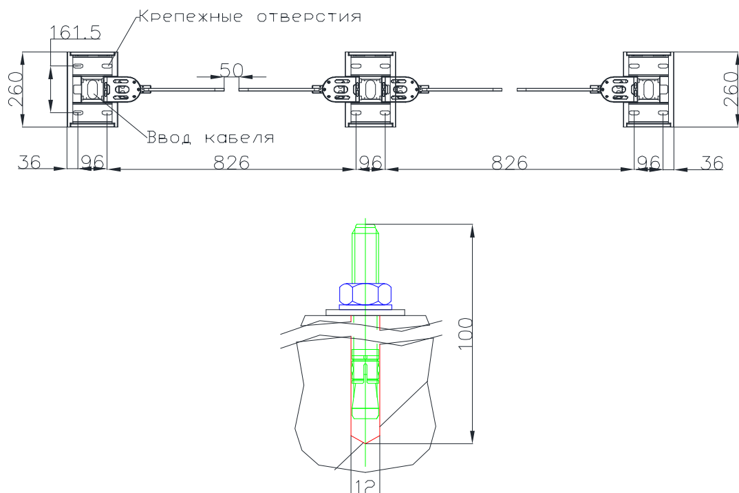
Рисунок 3 – Монтажные отверстия для дюбелей в нижней части тумбы
